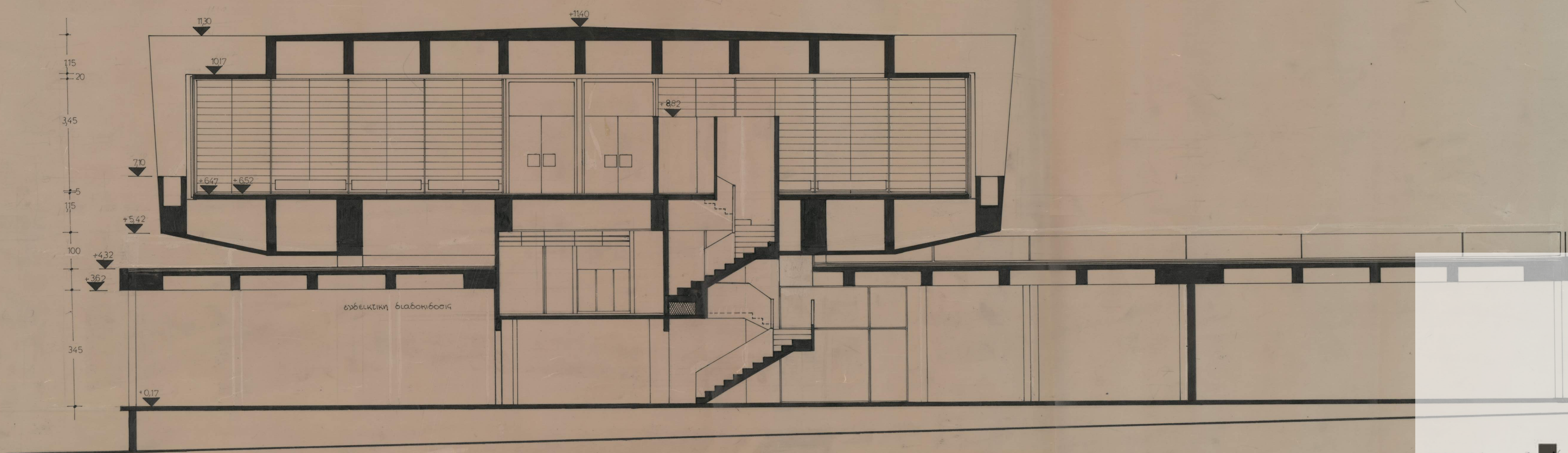
ΤΟΜΗ Α-Α'
