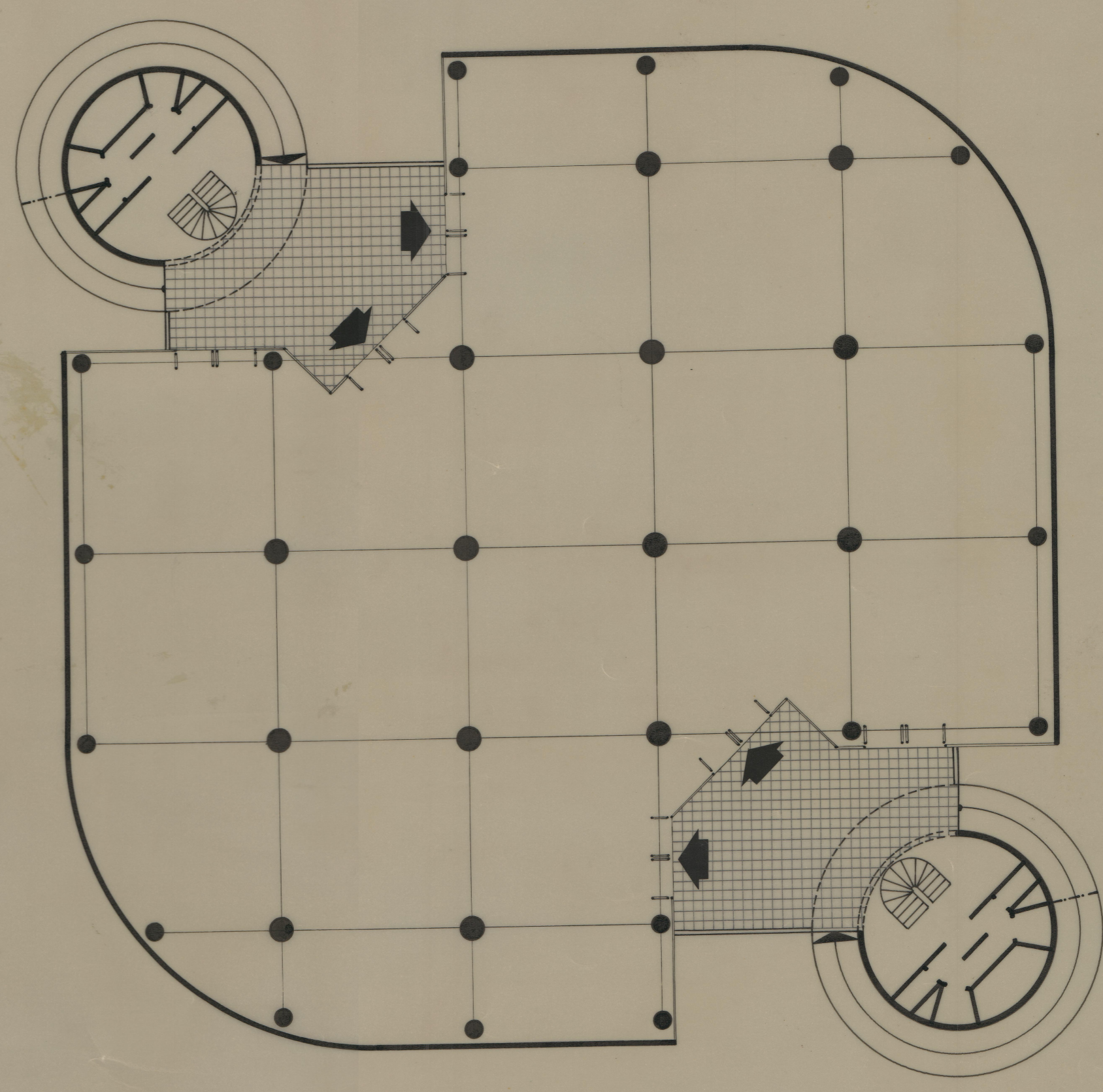
ΠΕΡΙΠΤΕΡΟ Α ΟΡΟΦΟΣ 1:200
