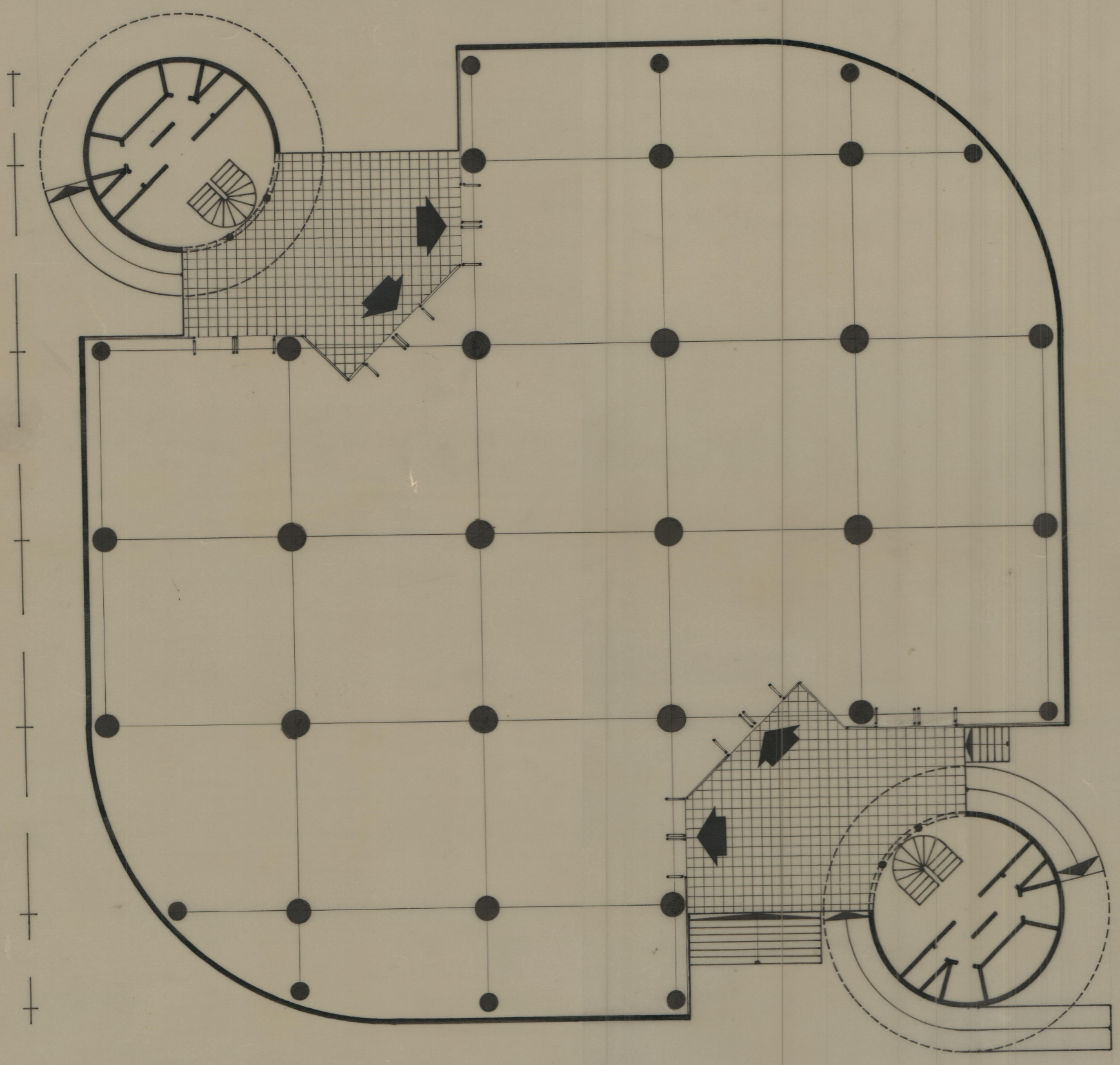
ΠΕΡΙΠΤΕΡΟ Α ΙΣΟΓΕΙΟ 1:200
